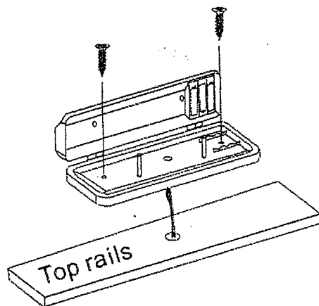
FIG 2: Fixer le compteur à la bande supérieure du plateau de la table à l'aide de deux vis.
